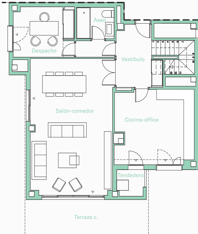
PLANTA INFERIOR
